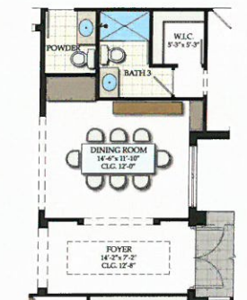
FORMAL DINING ROOM IN LIEU OF DEN OPTION
